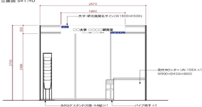
立面図 S=1:40
