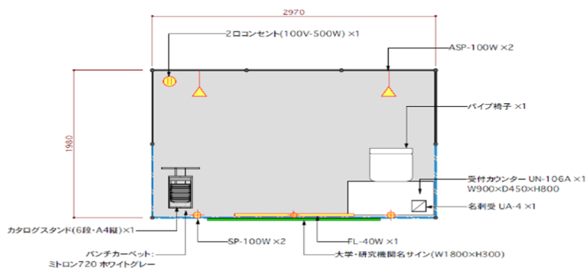
パッケージブース詳細図 S=1:40
