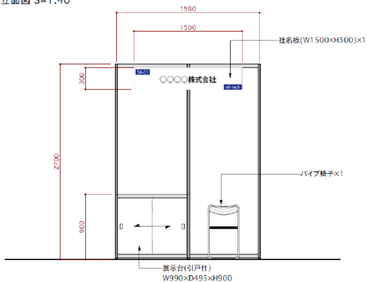
立面図 S=1:40
